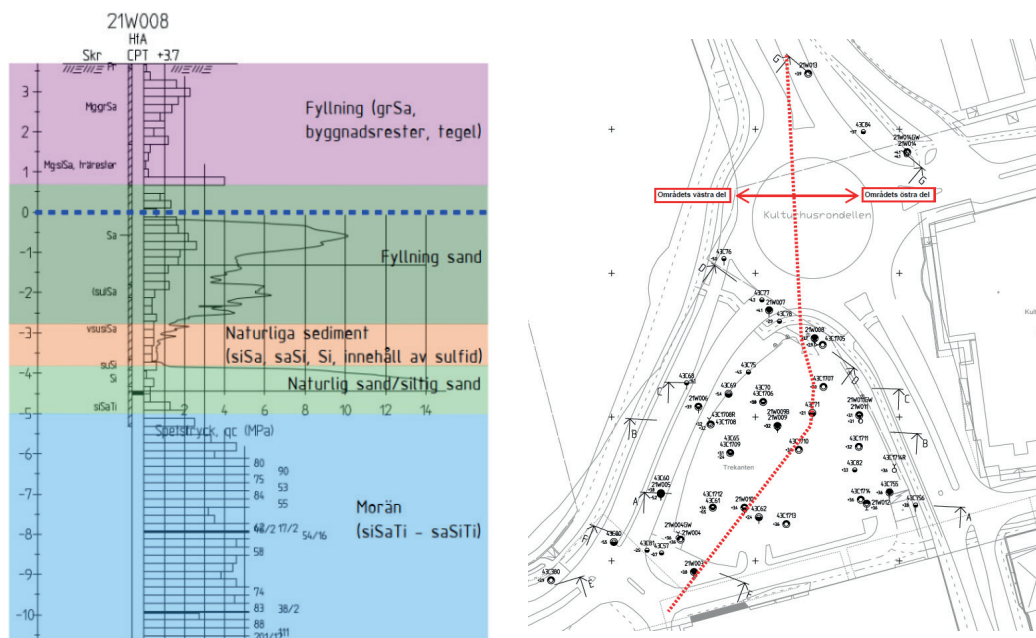
Figur 31 Principiell skiss över jordlagerföljden inom planområdet samt avgränsning av det västra och östra området (PM Geoteknik, WSP 2022)
