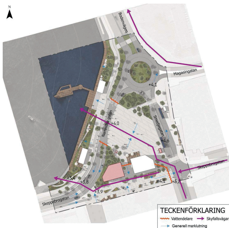
Figur 36 Översikt med förslag på sekundära avrinningsstråk vid skyfall illustrerade (Sweco, 2022).
