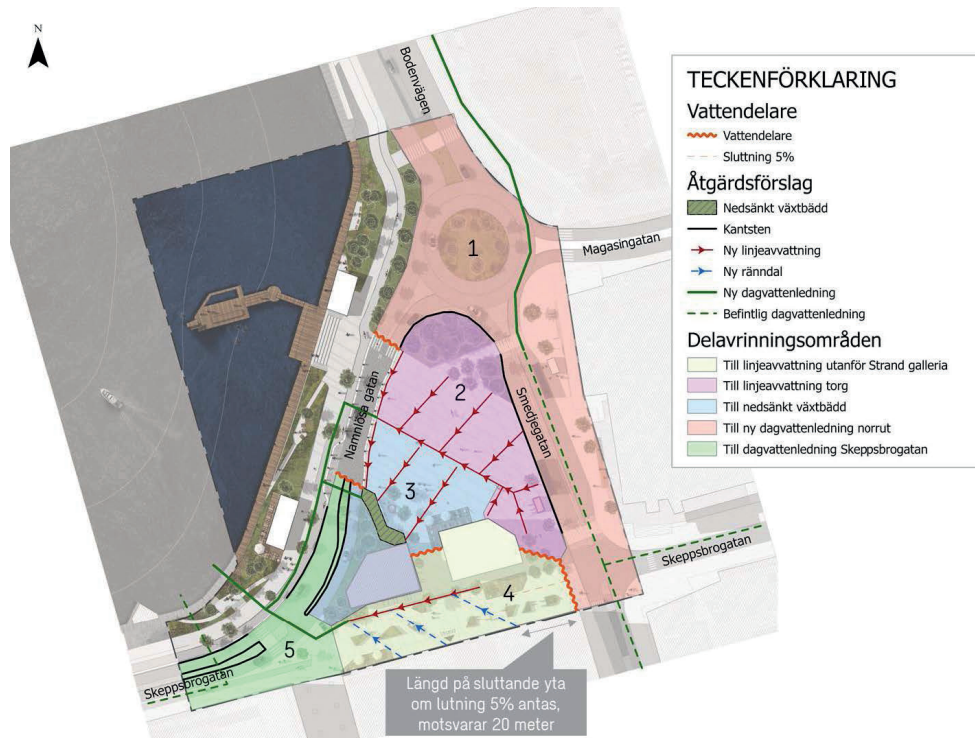
Figur 35 Förslag på systemhantering för dagvatten (Sweco, 2022).
